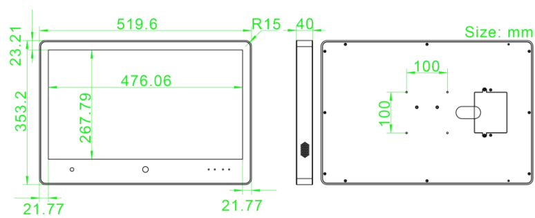
尺寸图
